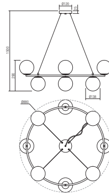
01-3159 Matt Gold 01-3160 Sand Black E14, 8 x max. 28W
