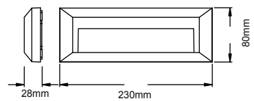
SLIM32*
