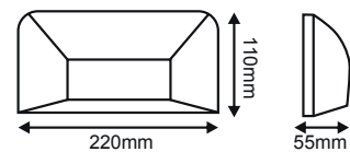
SLIM22*
