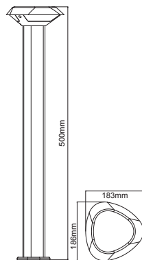
LG3802G-500
